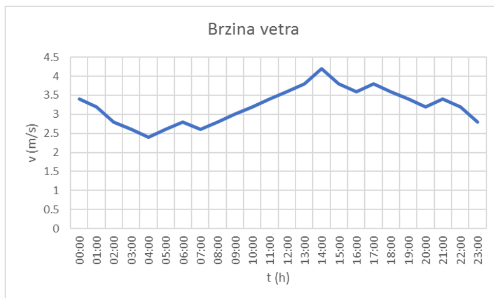
Slika 2.8. Brzina vetra tokom perioda merenja 23.02.2022. godine
