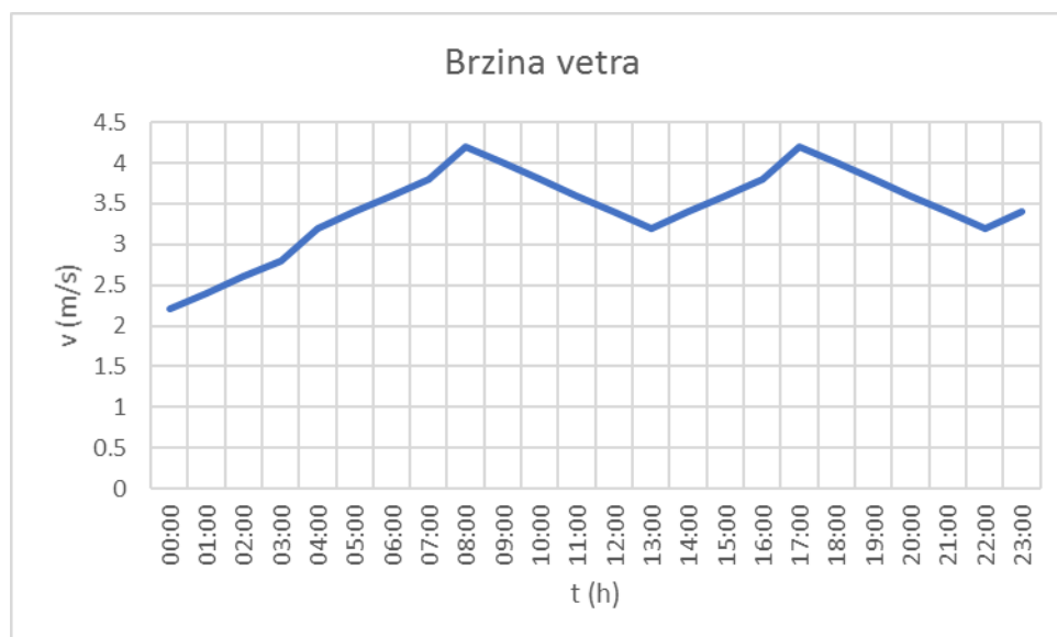
Slika 2.4. Brzina vetra tokom perioda merenja 22.02.2022. godine
