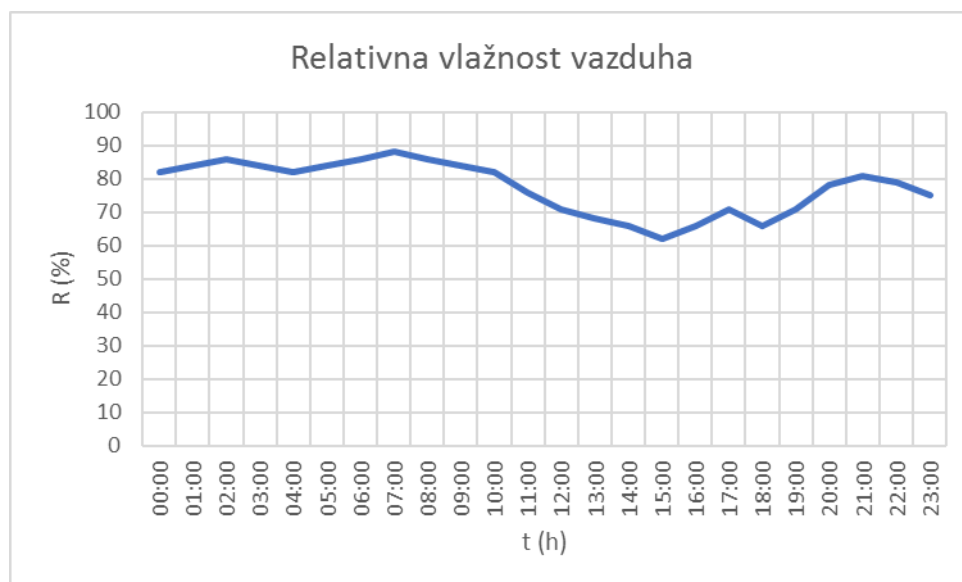
Slika 2.2. Relativna vlažnost vazduha tokom perioda merenja 22.02.2022. godine
