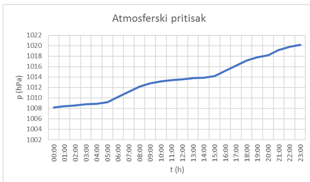
Slika 2.3. Atmosferski pritisak tokom perioda merenja 22.02.2022. godine
