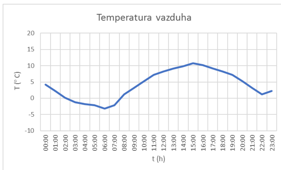
Slika 2.5. Temperatura vazduha tokom perioda merenja 23.02.2022. godine
