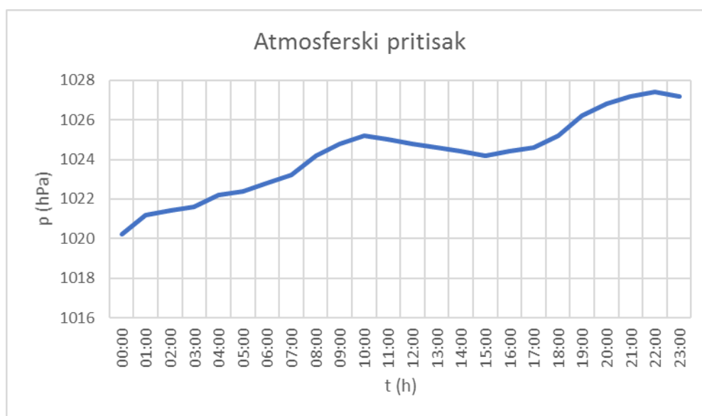
Slika 2.7. Atmosferski pritisak tokom perioda merenja 23.02.2022. godine
