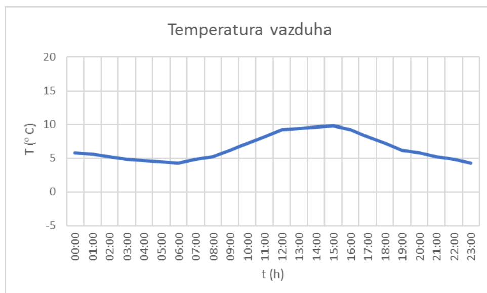
Slika 2.1. Temperatura vazduha tokom perioda merenja 22.02.2022. godine
