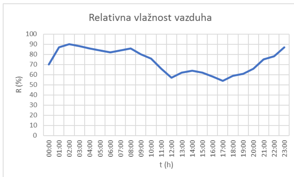
Slika 2.6. Relativna vlažnost vazduha tokom perioda merenja 23.02.2022. godine
