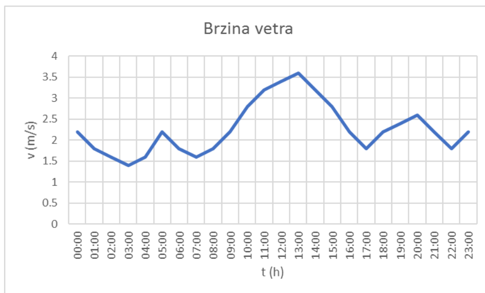
Slika 2.4. Brzina vetra tokom perioda merenja 25.01.2022. godine
