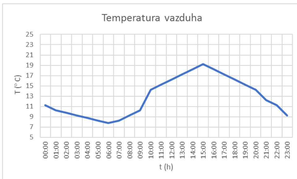
Slika 2.5. Temperatura vazduha tokom perioda merenja 28.10.2022. godine
