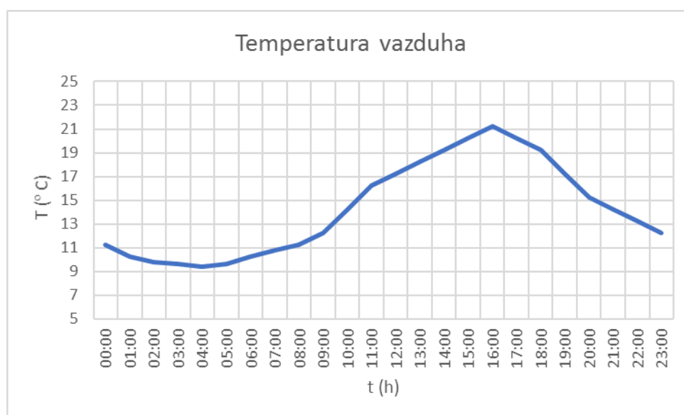
Slika 2.1. Temperatura vazduha tokom perioda merenja 27.10.2022. godine
