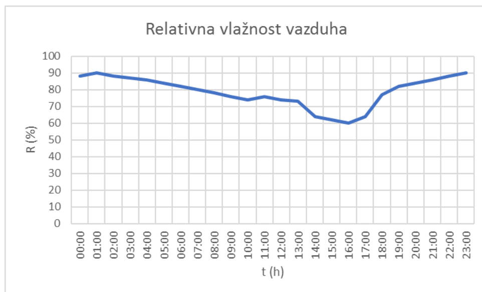
Slika 2.6. Relativna vlažnost vazduha tokom perioda merenja 28.10.2022. godine
