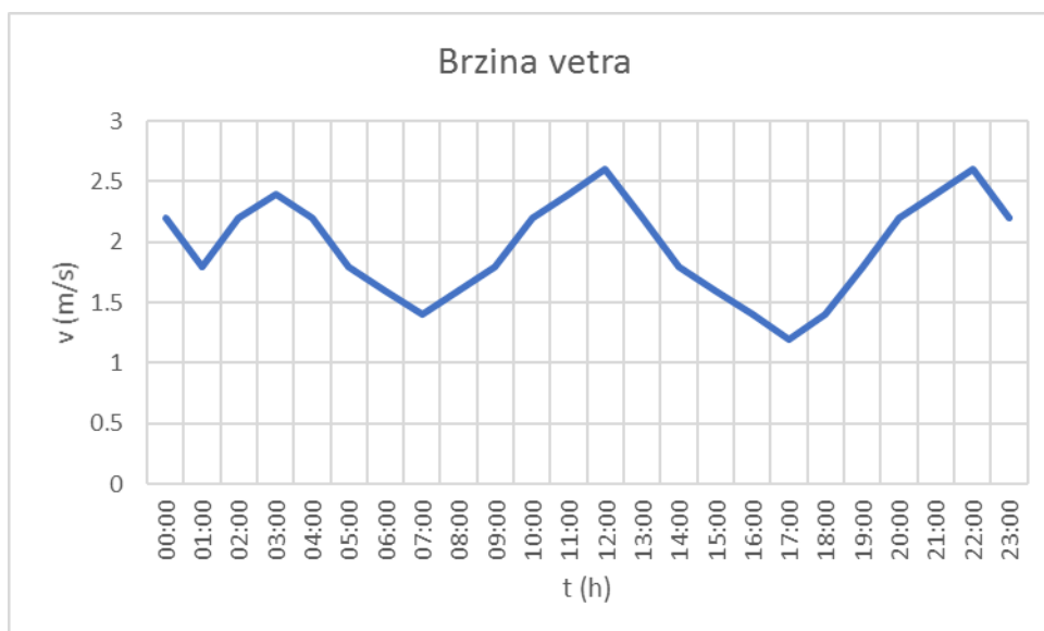
Slika 2.4. Brzina vetra tokom perioda merenja 27.10.2022. godine
