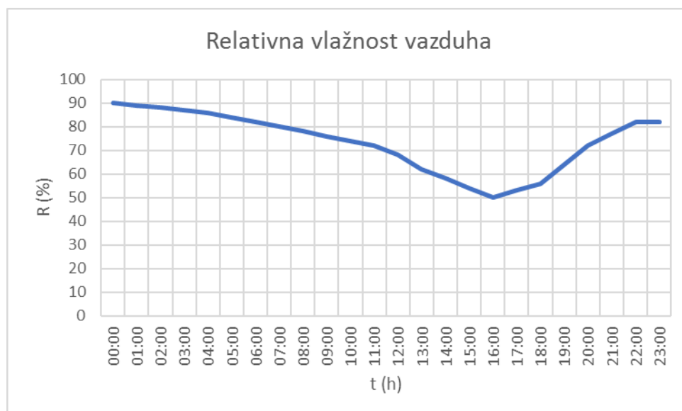
Slika 2.2. Relativna vlažnost vazduha tokom perioda merenja 27.10.2022. godine
