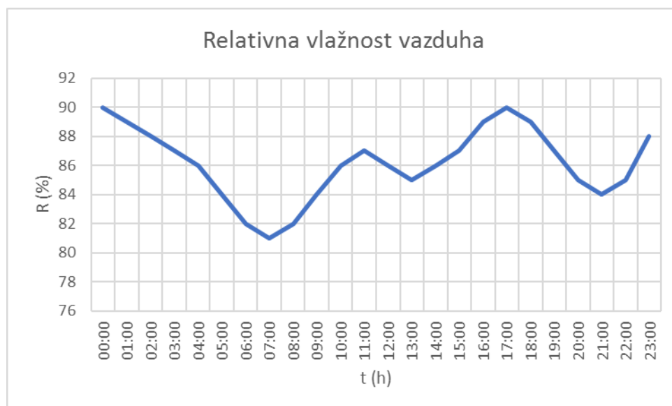
Slika 2.2. Relativna vlažnost vazduha tokom perioda merenja 27.09.2022. godine
