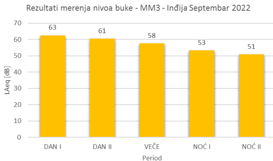
Slika 7.3. Rezultati merenja nivo buke MM3
