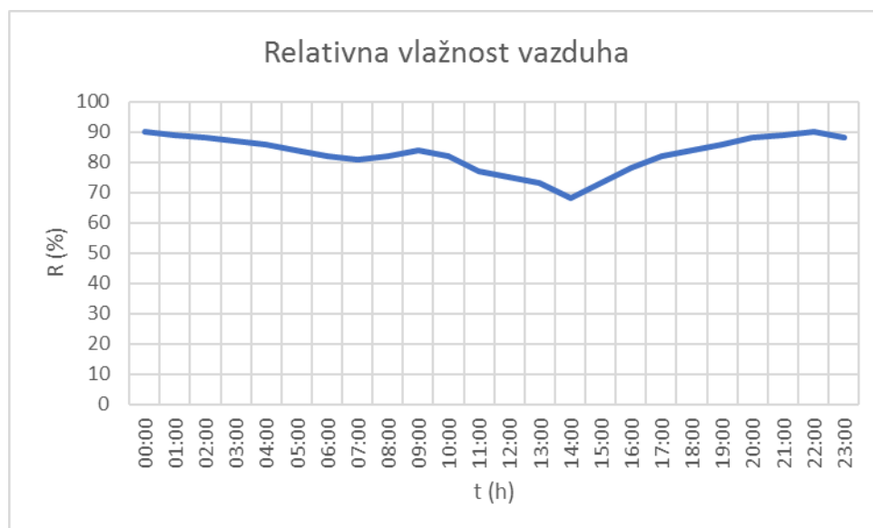
Slika 2.6. Relativna vlažnost vazduha tokom perioda merenja 28.09.2022. godine
