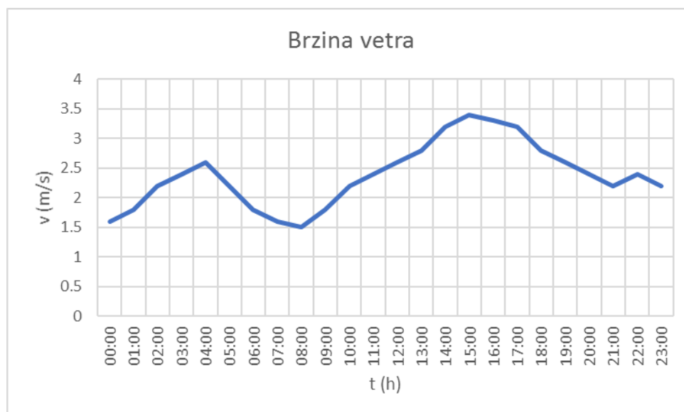
Slika 2.8. Brzina vetra tokom perioda merenja 28.09.2022. godine
