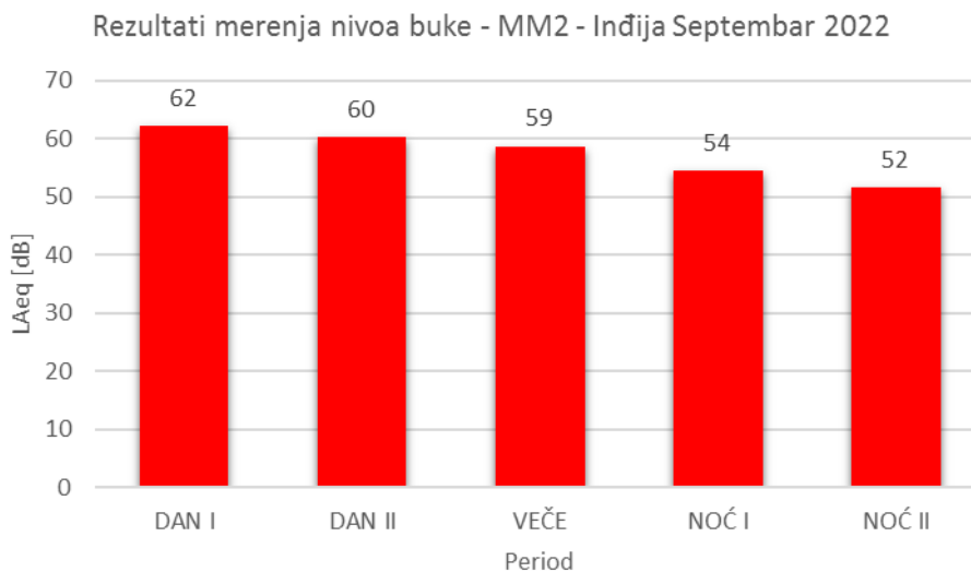
Slika 7.2. Rezultati merenja nivo buke MM2
