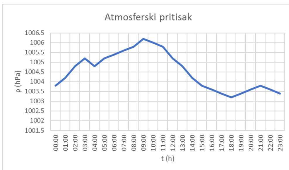
Slika 2.7. Atmosferski pritisak tokom perioda merenja 28.09.2022. godine
