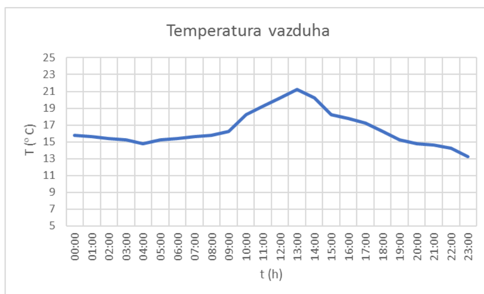
Slika 2.1. Temperatura vazduha tokom perioda merenja 27.09.2022. godine
