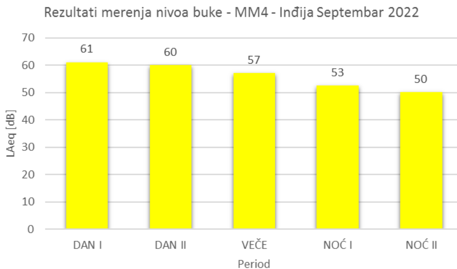
Slika 7.4. Rezultati merenja nivo buke MM4
