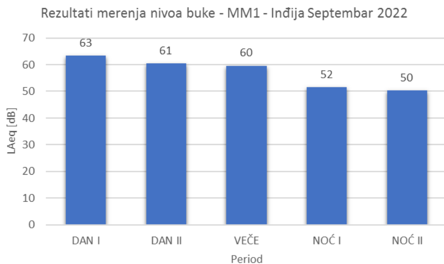
Slika 7.1. Rezultati merenja nivo buke MM1
