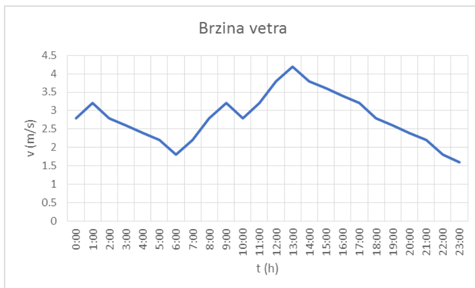
Slika 2.8. Brzina vetra tokom perioda merenja 27.04.2023. godine
