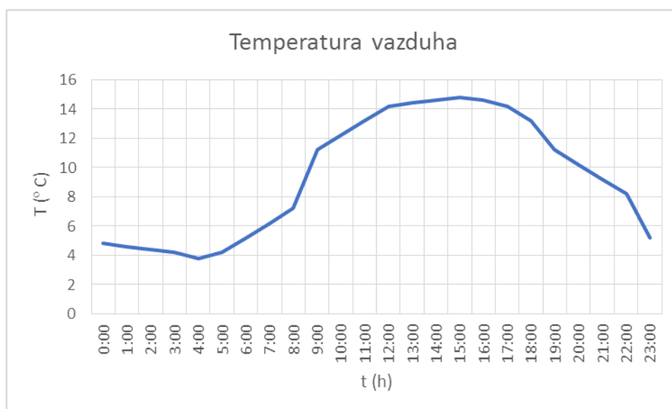
Slika 2.5. Temperatura vazduha tokom perioda merenja 27.04.2023. godine
