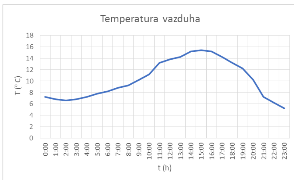
Slika 2.1. Temperatura vazduha tokom perioda merenja 26.04.2023. godine
