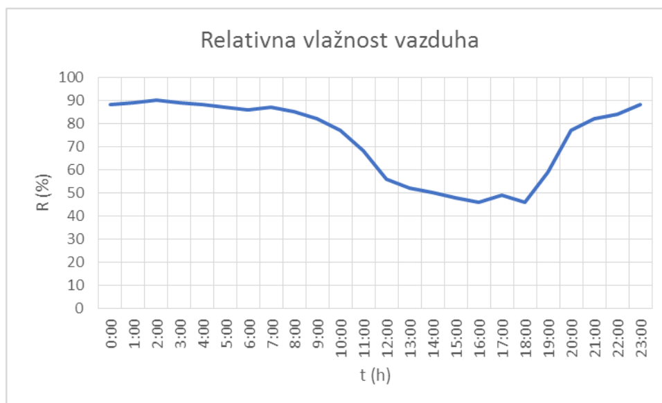
Slika 2.2. Relativna vlažnost vazduha tokom perioda merenja 26.04.2023. godine
