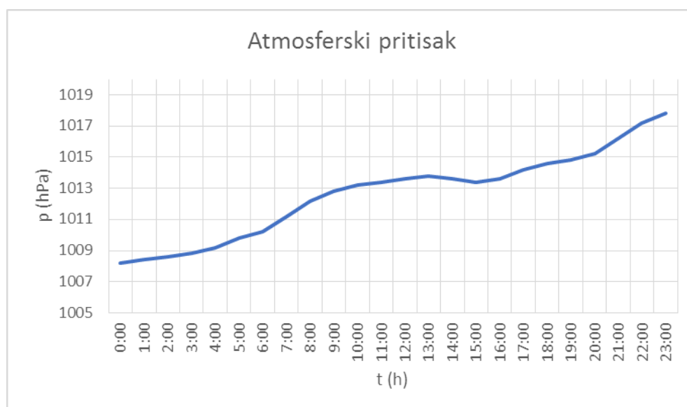
Slika 2.3. Atmosferski pritisak tokom perioda merenja 26.04.2023. godine
