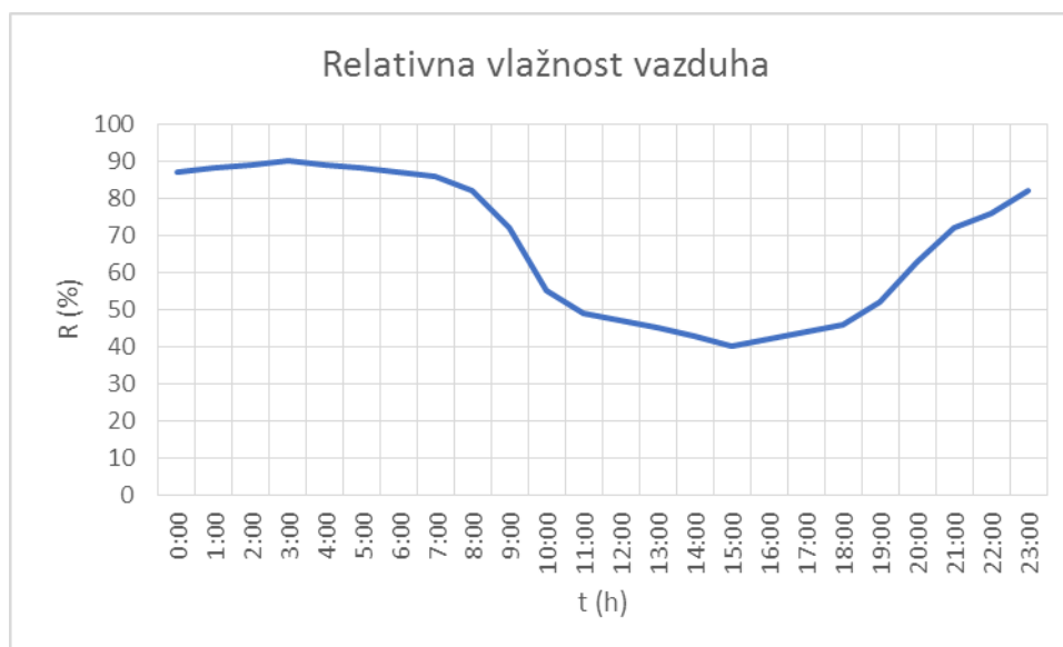
Slika 2.6. Relativna vlažnost vazduha tokom perioda merenja 27.04.2023. godine
