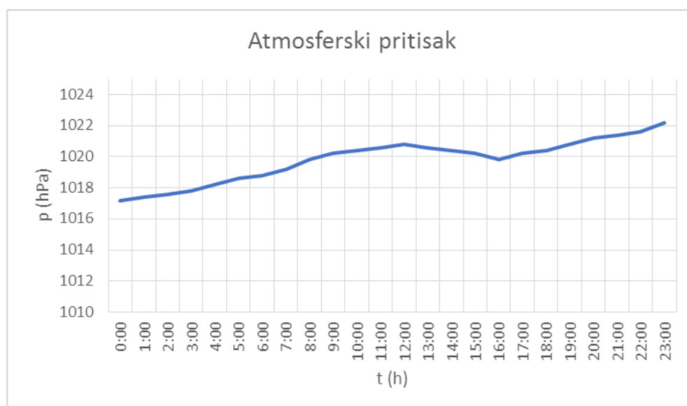
Slika 2.7. Atmosferski pritisak tokom perioda merenja 27.04.2023. godine
