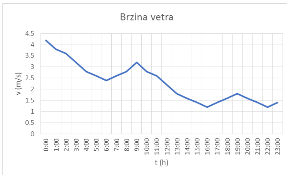
Slika 2.4. Brzina vetra tokom perioda merenja 26.04.2023. godine
