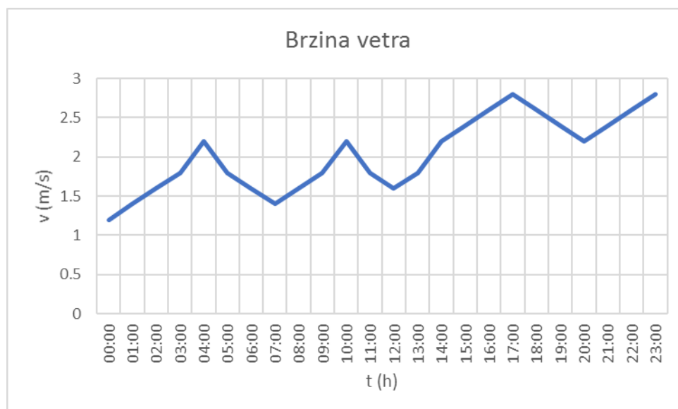
Slika 2.4. Brzina vetra tokom perioda merenja 17.07.2023. godine
