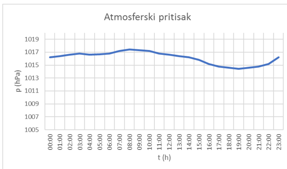
Slika 2.3. Atmosferski pritisak tokom perioda merenja 17.07.2023. godine
