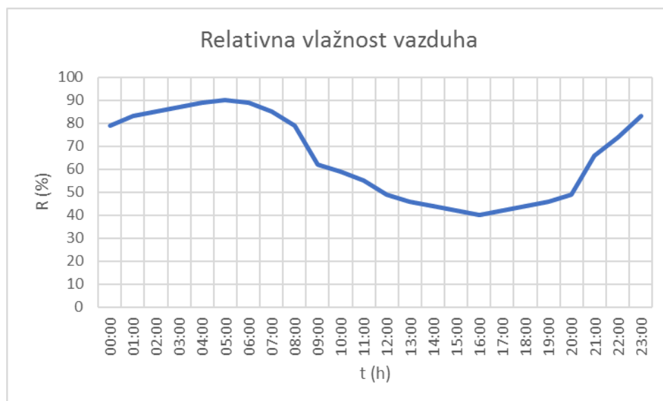
Slika 2.6. Relativna vlažnost vazduha tokom perioda merenja 18.07.2023. godine
