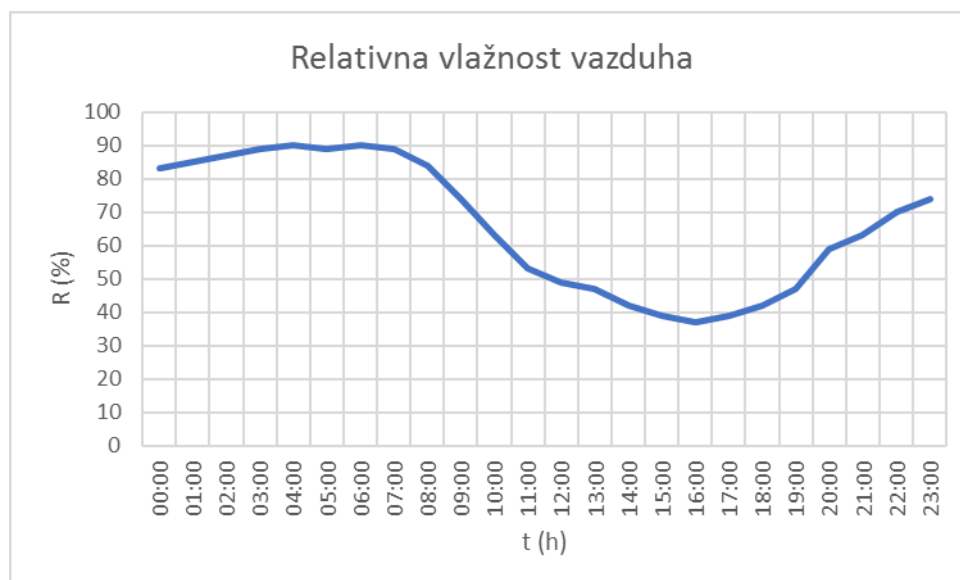
Slika 2.2. Relativna vlažnost vazduha tokom perioda merenja 17.07.2023. godine
